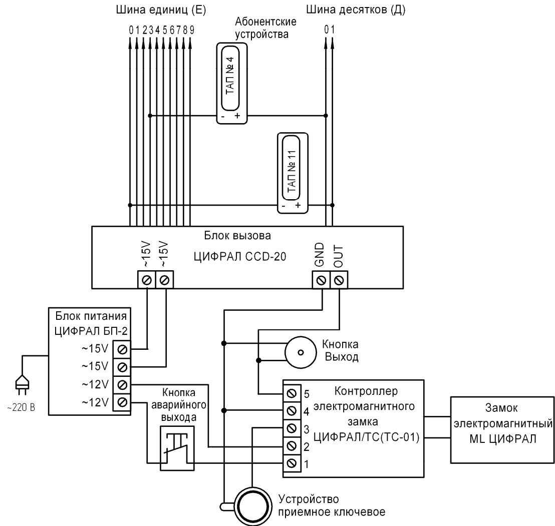
Рисунок Б.1 Схема подключения домофона ЦИФРАЛ ССD-20
