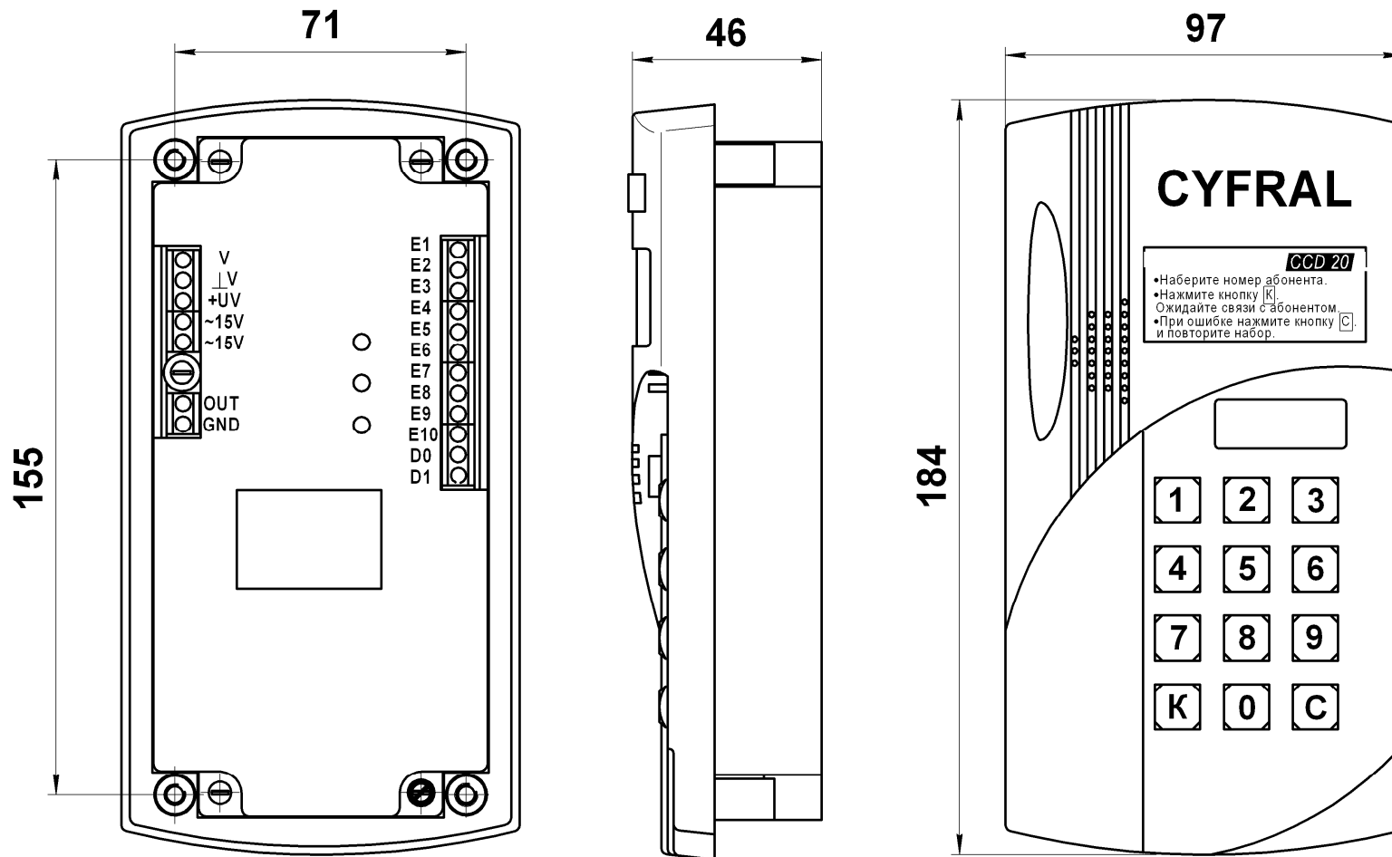
Рисунок А.1 Габаритные и установочные размеры блоков вызова ЦИФРАЛ ССD-20, ЦИФРАЛ ССD-20/V
