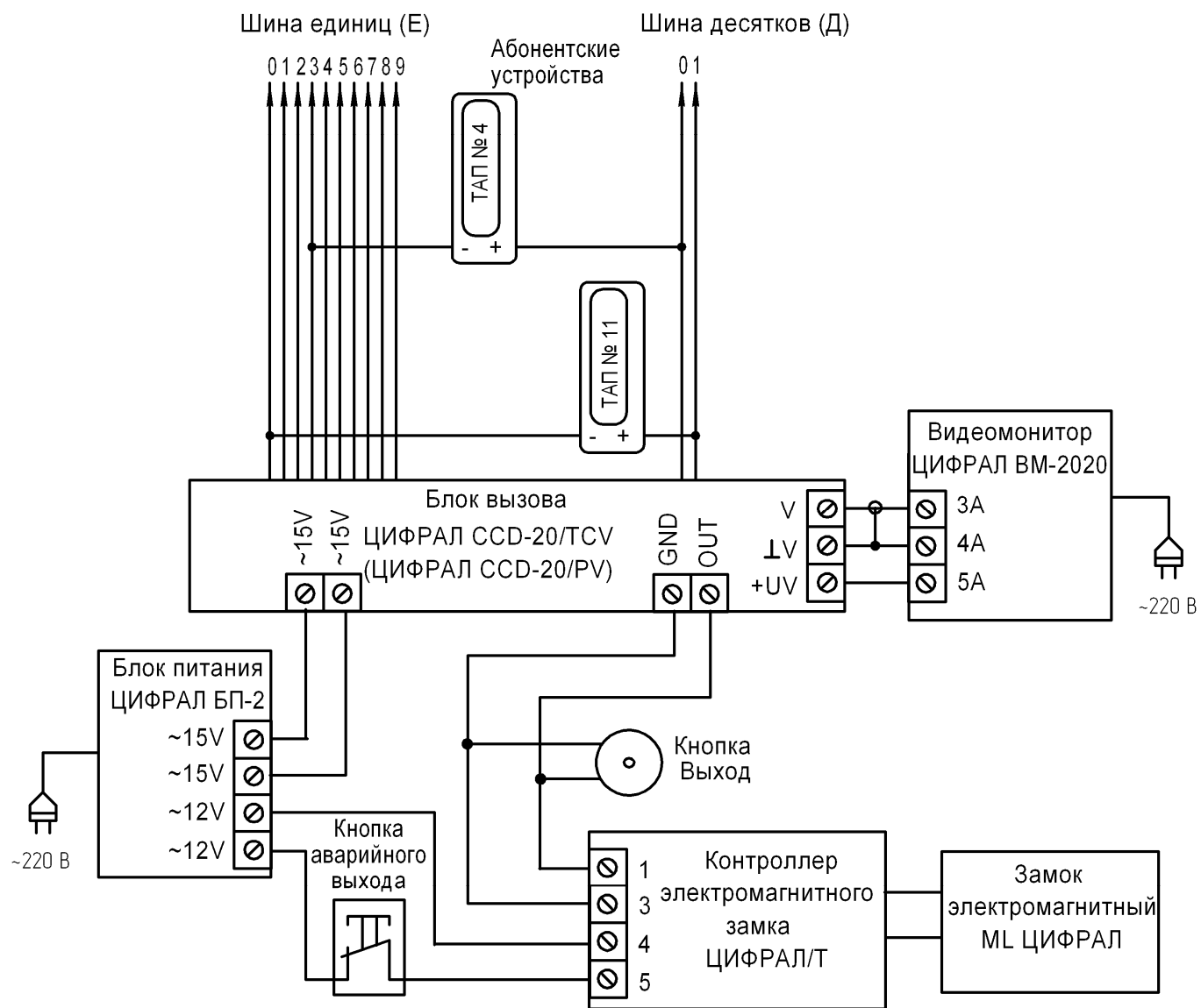
Рисунок Б.4 Схема подключения домофонов ЦИФРАЛ ССD-20/ТСV, ЦИФРАЛ ССD-20/PV
