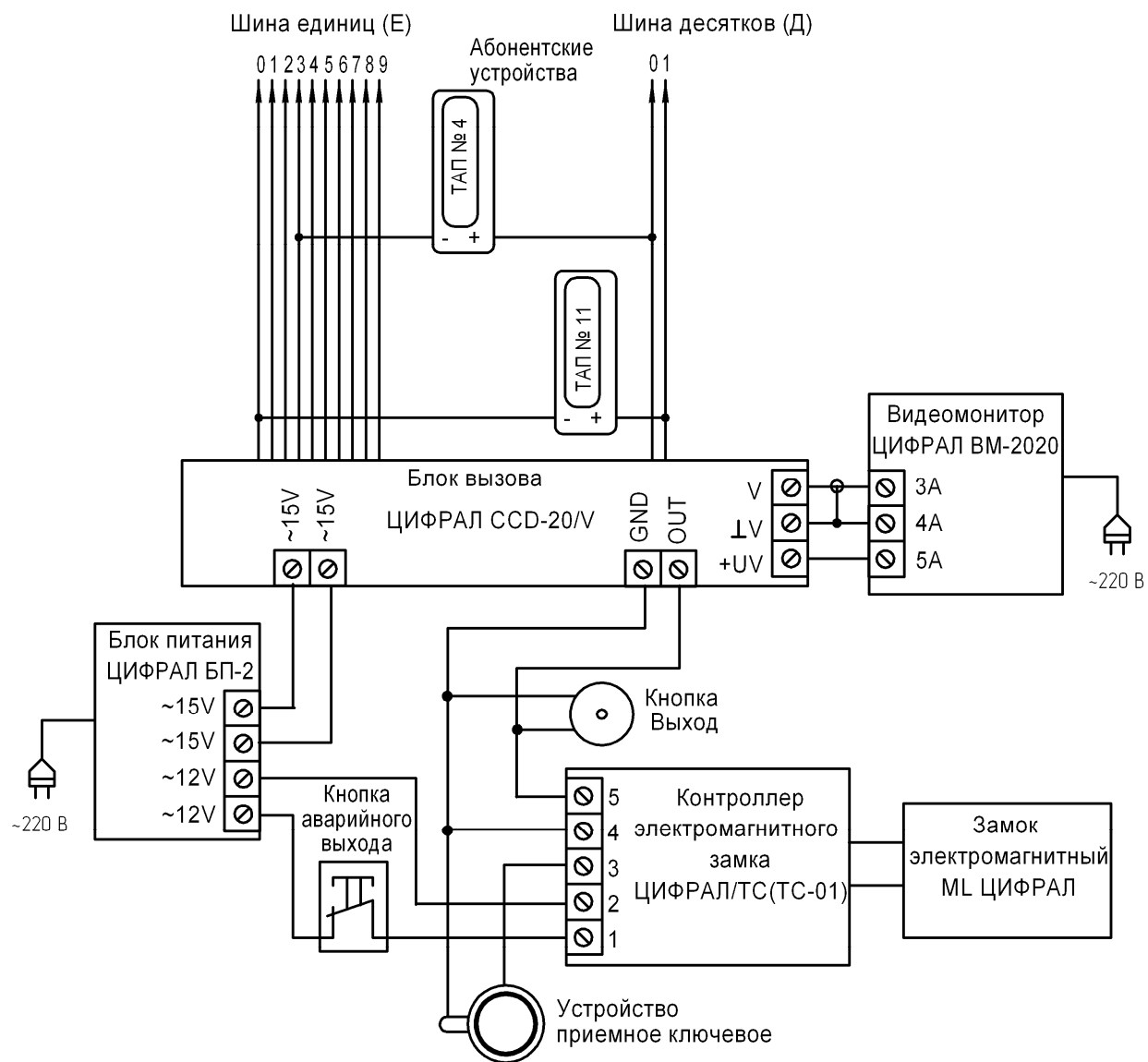
Рисунок Б.2 Схема подключения домофона ЦИФРАЛ ССД-20/V
